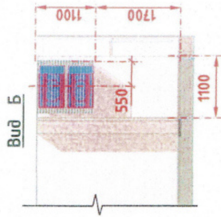
Эскиз элемента фасада с указанием места размещения оборудования
